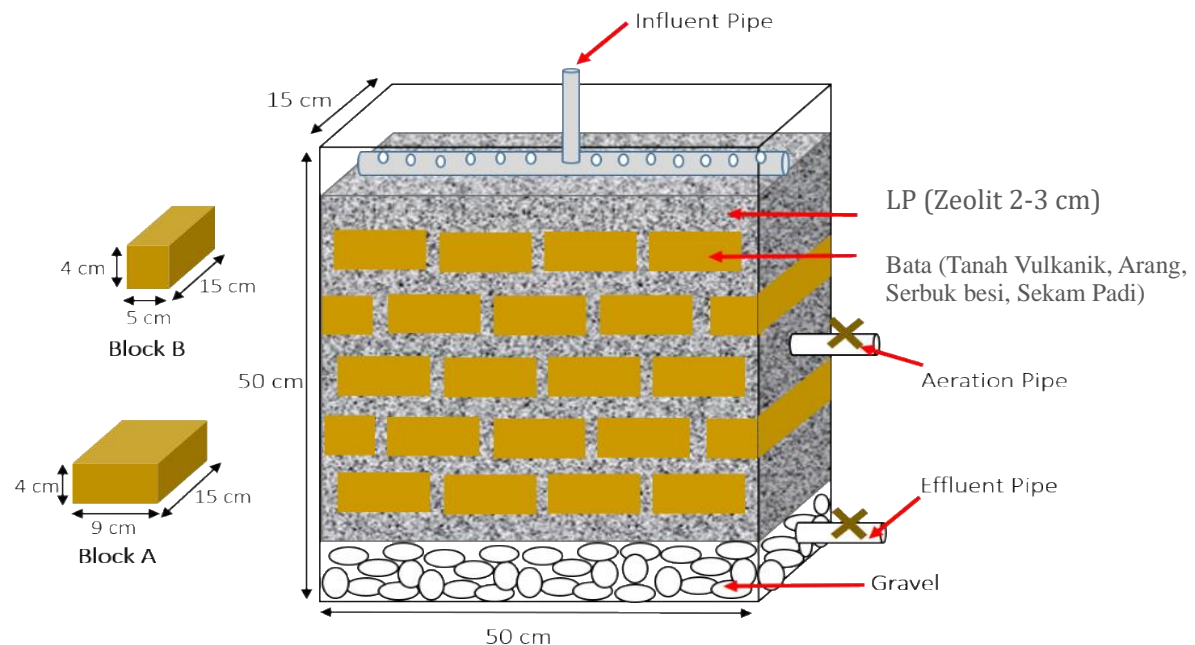
Gambar 1. Desain Reaktor LMM
